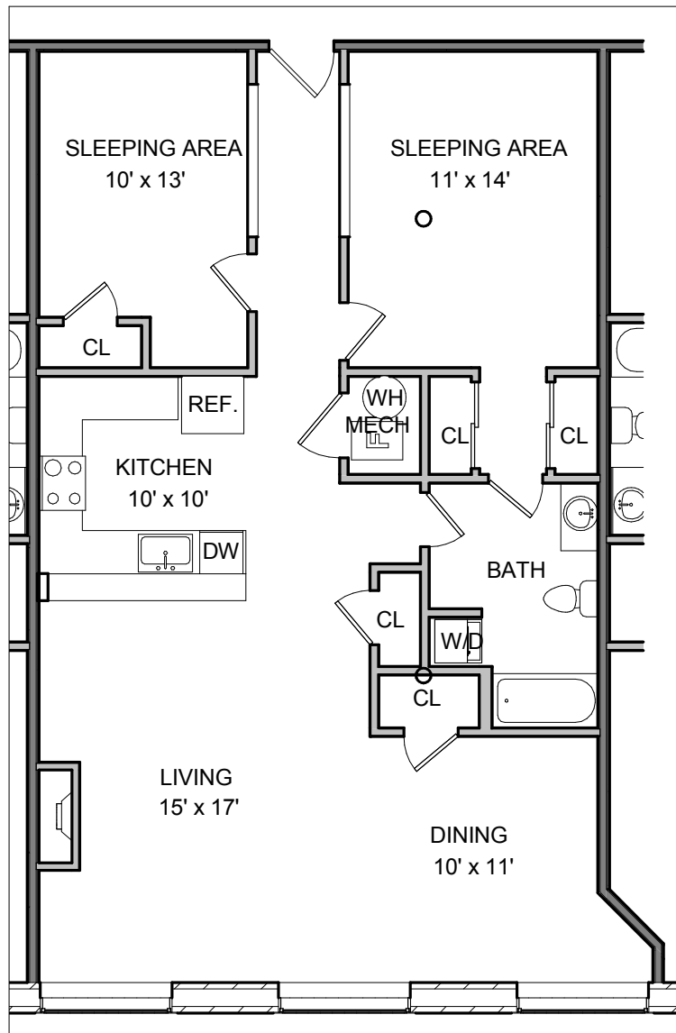
① D118 1/8" = 1'-0" SIMILAR TO UNIT D140 OPP. SIMILAR TO UNIT D139
